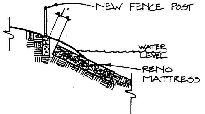
TYPICAL SECTION N.T.S.
